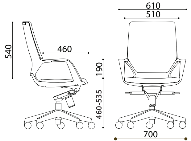
908*KTA72N2
